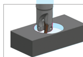
Interpolation hélicoïdale
