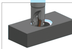
Interpolation d'alésage
